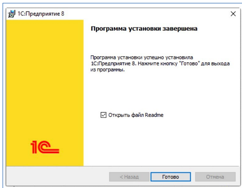
Рисунок 5 – Завершение установки
